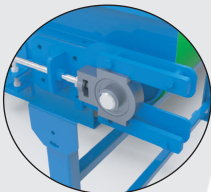
Chumacera Tensora para alinear y tensor banda
