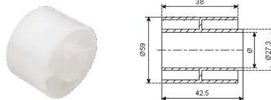
N418 托轮 N418 Roller
