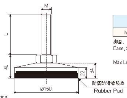
MFD150 金属固定调整脚踏 MFD150 Metal Fixed feet
