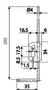
编号 (Code): N300 水槽吊架头 Head Of Drip Tray Supports 材质(Material): SUS304 Washer 不锈钢垫片 Clamp in Polyamide 尼龙夹
