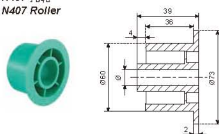
N407 托轮 N407 Roller
