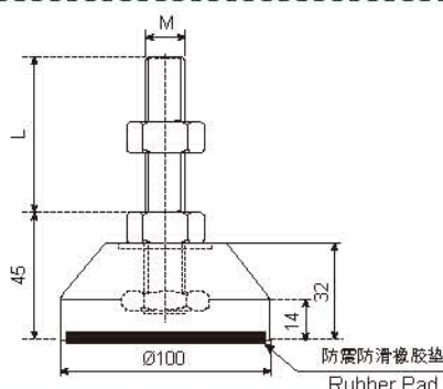
MFD100 金属固定调整脚踏 MFD100 Metal Fixed feet
