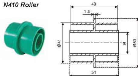
N410 托轮 N410 Roller
