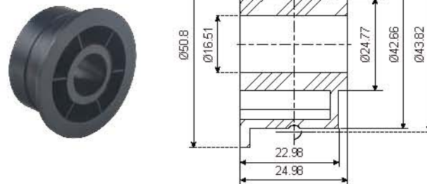
N418 托轮 N418 Roller
