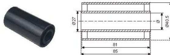
N420 托轮 N420 Roller
