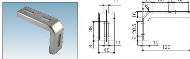
L 型不锈钢钣金支架 L Shape SS Brackets
