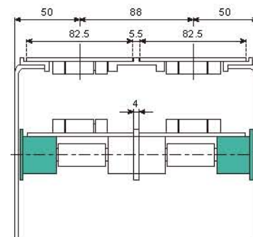
N414 托轮 N414 Roller
