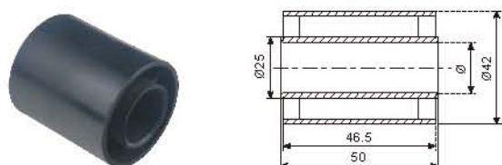
N419 托轮 N419 Roller
