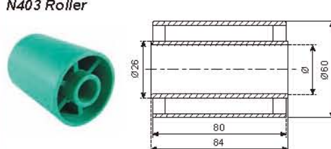
N403 托轮 N403 Roller
