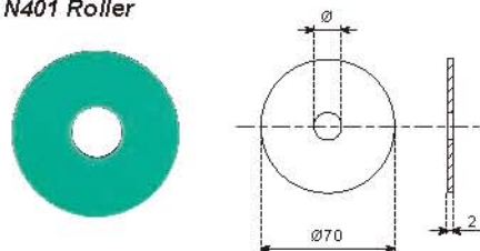
N401 托轮 N401 Roller
