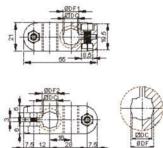
N201 小十字承夹 N201 Cross Clamps
