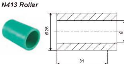
N413 托轮 N413 Roller
