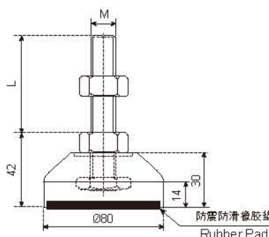
MFD80 金属固定调整脚踏 MFD80 Metal Fixed feet
