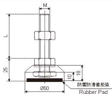
MFD50 金属固定调整脚踏 MFD50 Metal Fixed feet
