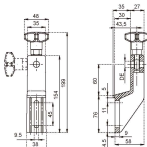
N240A 护栏支架 N240A Side Guide Brackets
