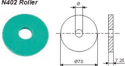
N402 托轮 N402 Roller
