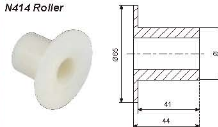
N414 托轮 N414 Roller
