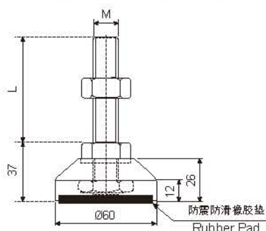
MFD60 金属固定调整脚踏 MFD60 Metal Fixed feet
