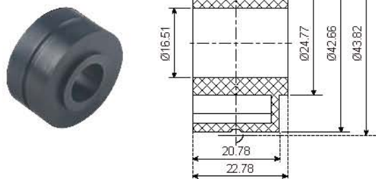
N417 托轮 N417 Roller
