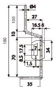
水槽吊架 Drip Tray Supports 材质(Material): SUS304 Supports 不锈钢吊钩 Clamp in Polyamide 尼龙夹
