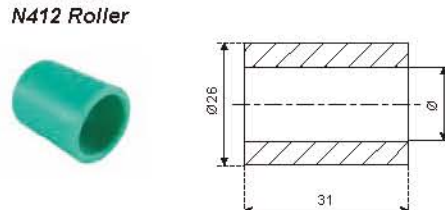
N412 托轮 N412 Roller
