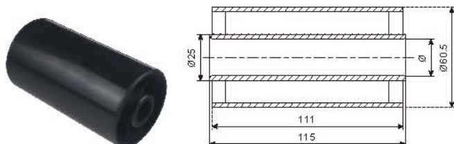
N421 托轮 N421 Roller
