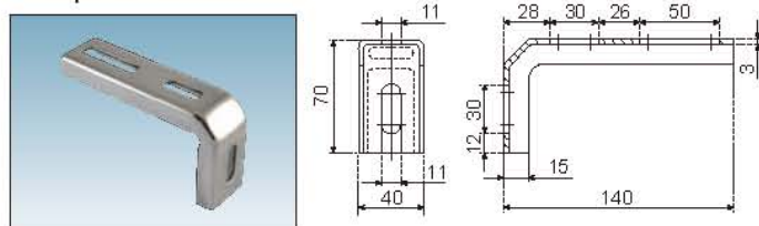
L 型不锈钢钣金支架 L Shape SS Brackets
