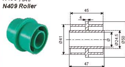
N409 托轮 N409 Roller
