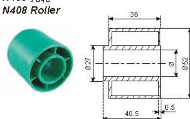
N408 托轮 N408 Roller
